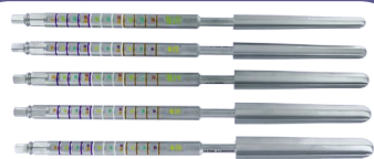
H28 001 to/à H28 005 Ø10 to 18mm Intramedullar reamer Alésoir intramédullaire
