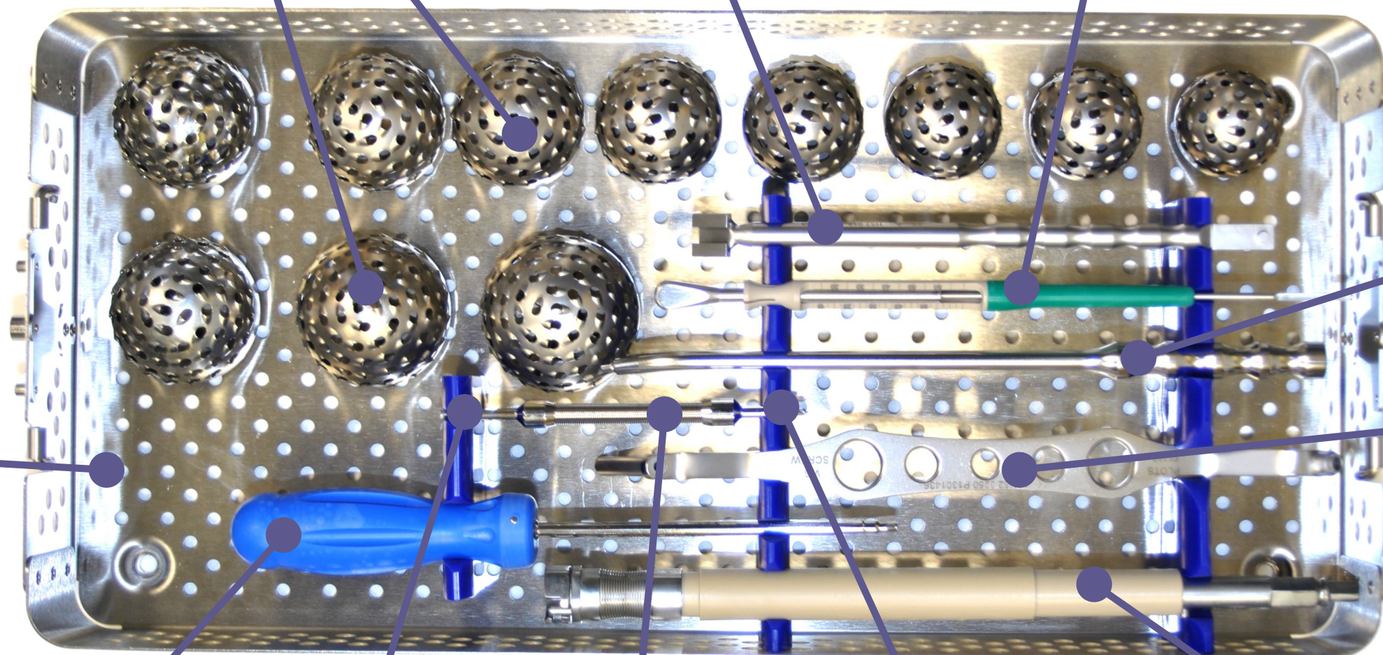
16-14-045 to 16-14-065 Acetabular reamers Ø 45 to 65 Fraises à cotyles Ø 45 à 65
