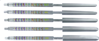
H28 001 to/à H28 005 Ø10 to 18mm Intramedullar reamer Alésoir intramédullaire
